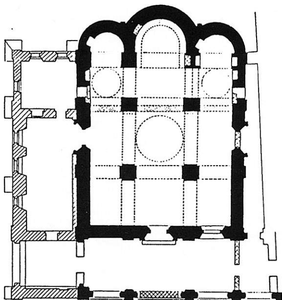
Ил. 1. План Спасского собора ярославского Спасо-Преображенского монастыря, сделанный реставратором И.М. Гудковым. По изд. 2002 г.
