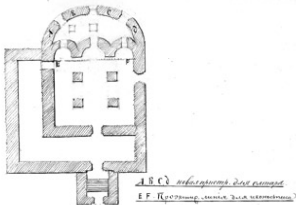
Ил. 1. План Спасского собора ярославского Спасо-Преображенского монастыря, сделанный реставратором И.М. Гудковым. По изд. 2002 г.
