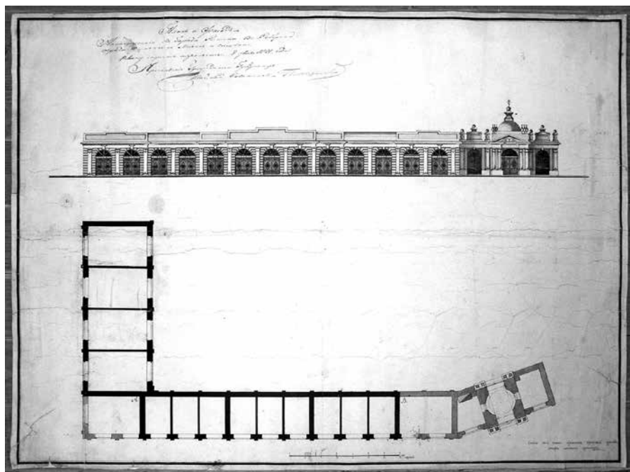
Ил. 5. Пракин М. «План и фасад на построение в городе Ростове в соборной ограде каменных лавок и часовни». 1831 г. ГМЗРК. Ар-259
