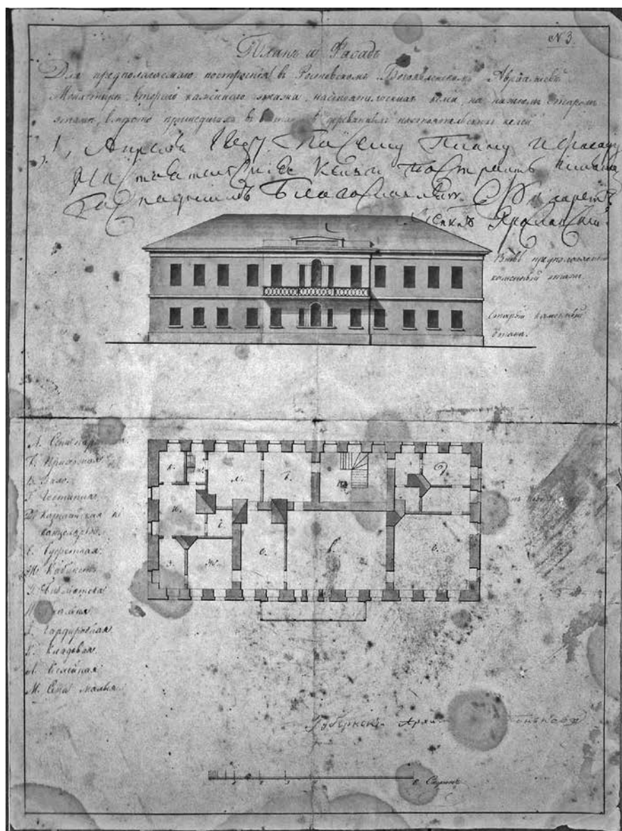
Ил. 11. Паньков П.Я. «План и фасад для предполагаемого построения в Ростовском Богоявленском Авраамиеве монастыре второго этажа настоятельских келей на нижнем старом этаже вместо пришедших в ветхость деревянных настоятельских келей». Около 1837 г. ГМЗРК. Ар-156
