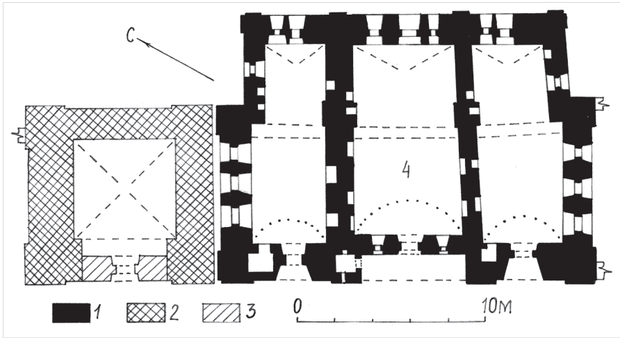
Ил. 1. План нижнего яруса соборной звонницы в Ростове. Обмер 1993 г. Из ст.: Мельник А. Г. Новое о звоннице // СРМ. Соборная звонница Ростова Великого. Ростов, 1993. С. 8. 1 – кладка около 1682 г.; 2 – кладка около 1688 г.; 3 – кладка конца XVII – начала XVIII в.; 4 – церковь Входа в Иерусалим
