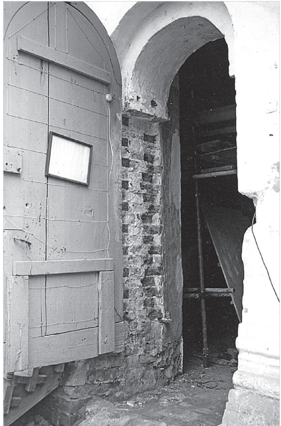
Ил. 22. Интерьер церкви Входа в Иерусалим соборной звонницы. Гнездо для балки хоров, устроенных в 2004 г. Фото 2004 г.
