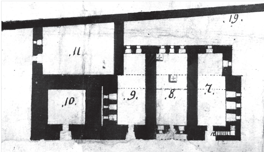
Ил. 2. План соборной звонницы в Ростове. Фрагмент плана Ростовского архиерейского двора 1793 г. Российская национальная библиотека
