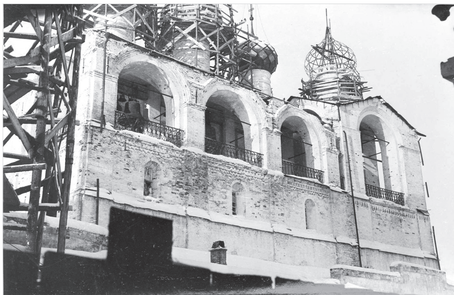
Ил. 20. Верхняя часть соборной звонницы в процессе реставрации. Вид с юго-востока. Фото 1955 г.
