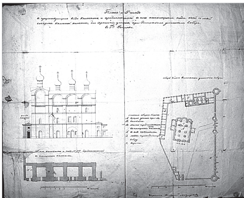
Ил. 6. План и фасад соборной звонницы с проектируемой северной пристройкой для хранения угля (№ 1) и план соборного двора. Середина XIX в. ГМЗРК
