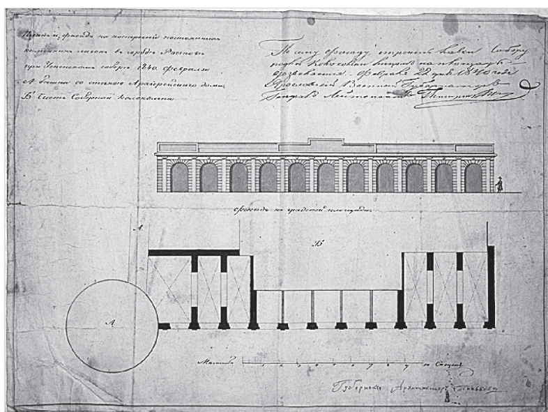
Ил. 5. Проект лавок, которые примкнули с востока, севера и юга к соборной звоннице. 1840 г. ГМЗРК
