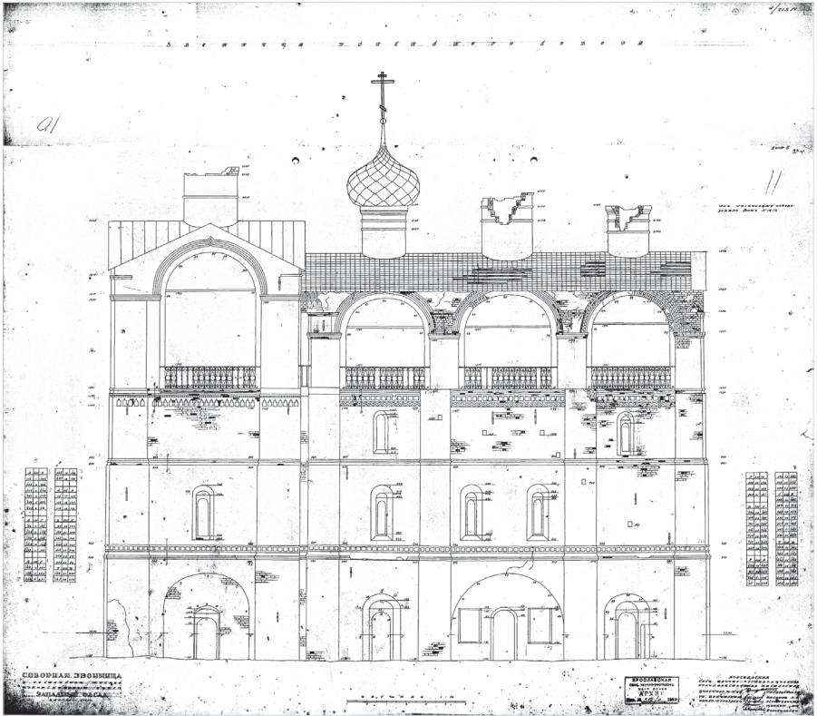
Ил. 15. Западный фасад соборной звонницы. Обмер 1955 г. ГМЗРК
