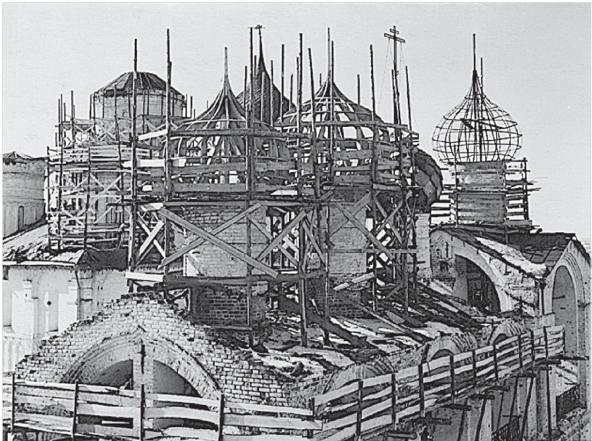
Ил. 19. Верхняя часть соборной звонницы в процессе реставрации. Вид с юго-востока. Фото 1955 г.
