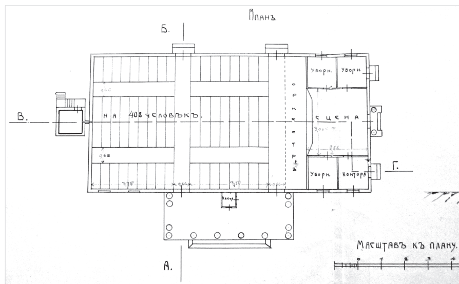
Ил. 2. Внутренняя планировка здания электротeatра в Городском саду, выполнена 24 марта 1914 г. гражданским архитектором Н. Ю. Лермонтовым (РФ ГАЯО. Ф. 2. Оп. 1. Д. 1101. Л. 18а)
