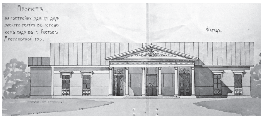
Ил. 1. Проект фасада здания электротeatра в Городском саду, выполнен 24 марта 1914 г. гражданским архитектором Н. Ю. Лермонтовым (РФ ГАЯО. Ф. 2. Оп. 1. Д. 1101. Л. 18а)
