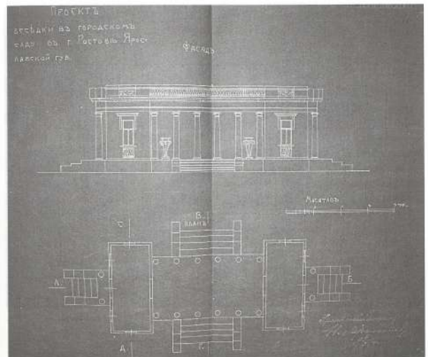
Илл. 3. Лермонтов Н. Проект беседки в городском саду. 1914. РФ ГАЯО. Ф. Р-1333. Оп. 1. Д. 13. л. 16.
