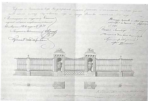
Илл. 2. Паньков П.Я. Чертеж в детальном виде на устройство железной решетки с каменными столбами общественного сада в г. Ростове. 1835. РФ ГАЯО. Ф. Р-1333. Оп. 1. Д. 13.
