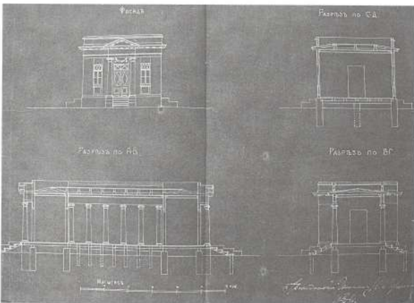
Илл. 4. Лермонтов Н. Проект беседки в городском саду. 1914. РФ ГАЯО. Ф. Р-1333. Оп. 1. Д. 13. л. 17
