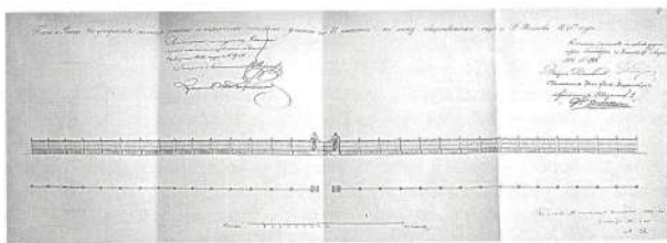
Илл. 1. Паньков П.Я. План и фасад на устройство железной решетки с каменными столбами общественного сада в г. Ростове. 1835. РФ ГАЯО, ф. Р-1333. Оп. 1. Д. 13.
