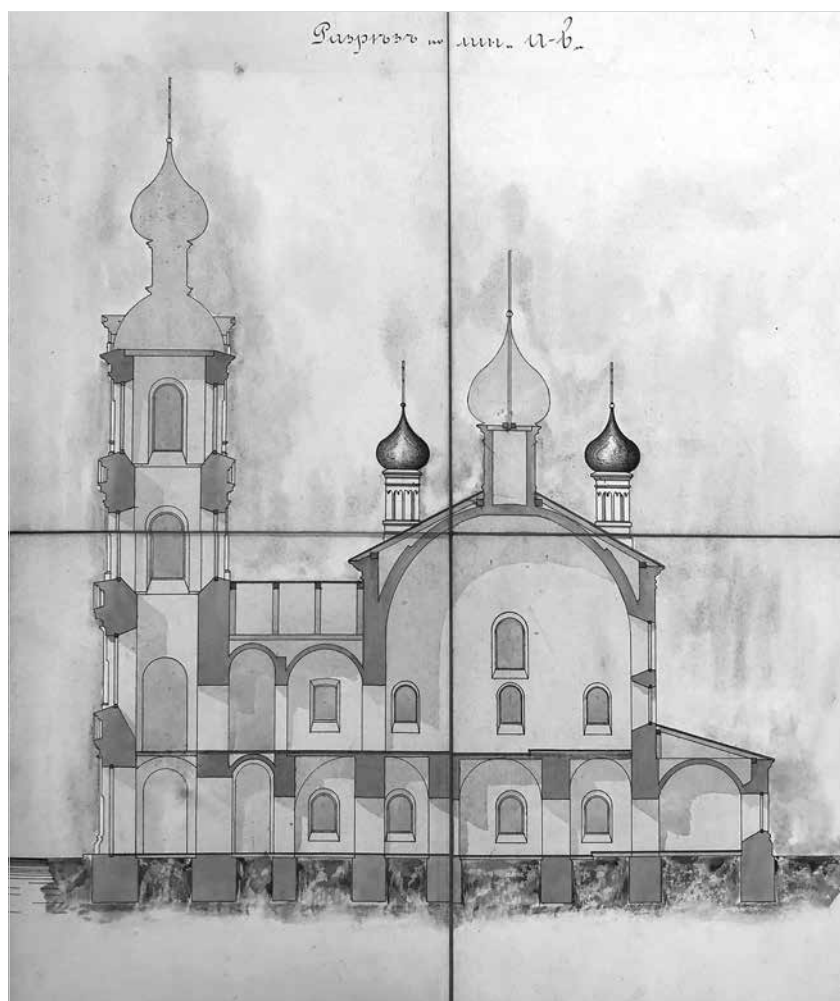
Ил. 4. Фрагмент чертежа церкви Казанской Божией Матери: разрез по линии а-в
