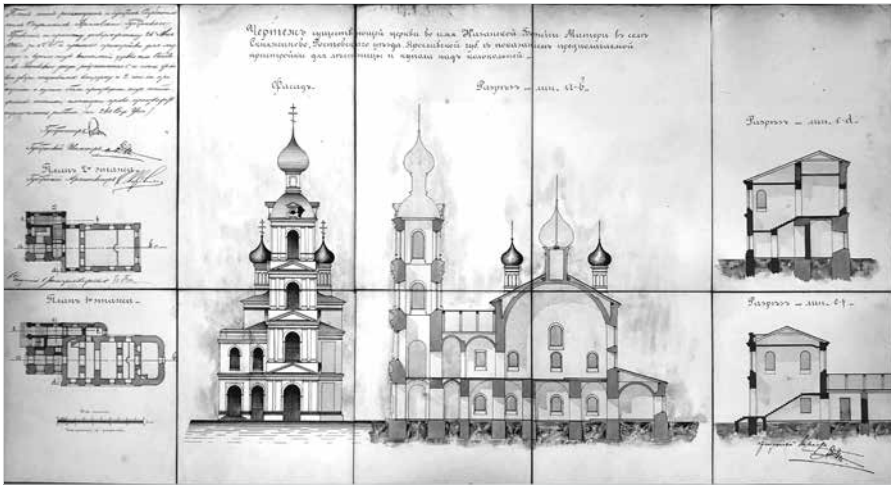
Ил. 1. Чертеж существующей церкви во имя Казанской Божией Матери в селе Скнятино, Ростовского уезда, Ярославской губ. с показанием предполагаемой пристройки для лестницы и купола над колокольней
