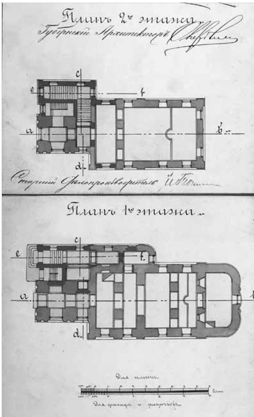
Ил. 1. Чертеж существующей церкви во имя Казанской Божией Матери в селе Скнятино, Ростовского уезда, Ярославской губ. с показанием предполагаемой пристройки для лестницы и купола над колокольней
