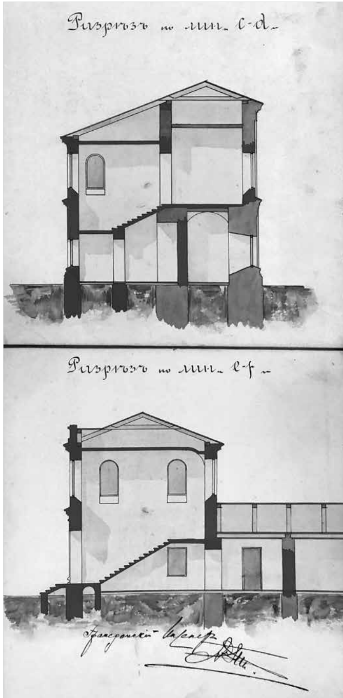
Ил. 4. Фрагмент чертежа церкви Казанской Божией Матери: разрезы по линиям с-д и е-ф (см. ил. 2)
