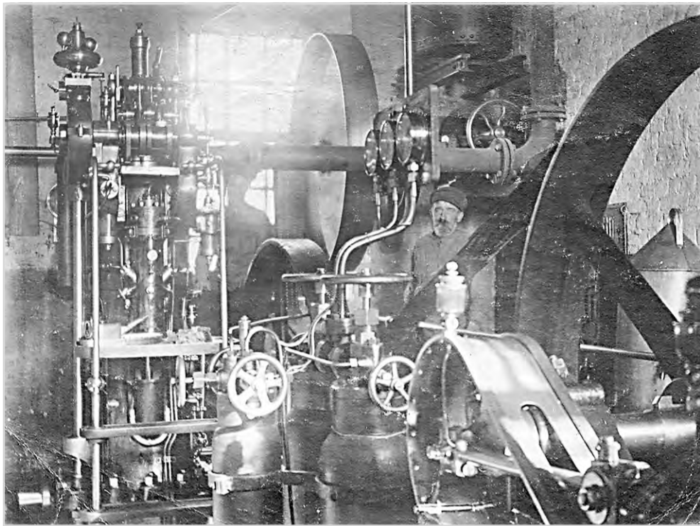
Ил. 2. Внутреннее устройство машинного отделения. На втором плане – обслуживающий персонал. Фото 1912 г.
