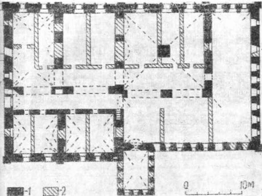
Рис. 2. План второго этажа комплекса Георгиевской церкви: 1 — кладка (1683 — после 1685 г.); 2 — кладка XIX—XX вв.
