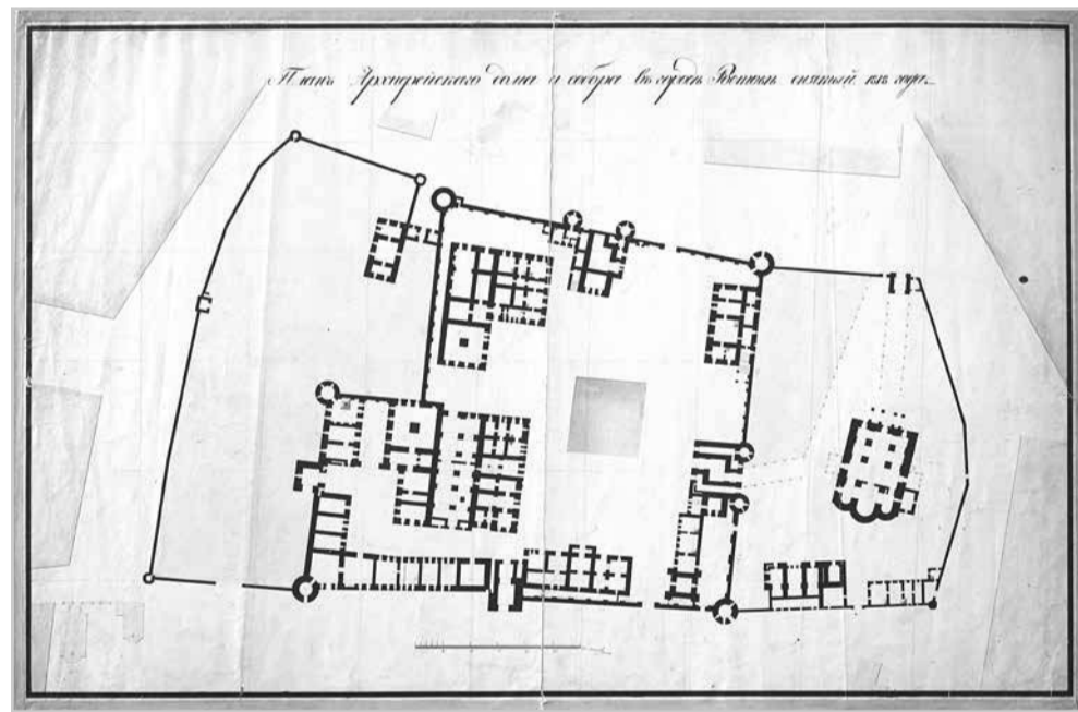
Ил. 8. Чертеж плана Ростовского кремля. 1830-е гг. Копия с чертежа П. Я. Панькова 1818 г. ГМЗРК. АР-117
