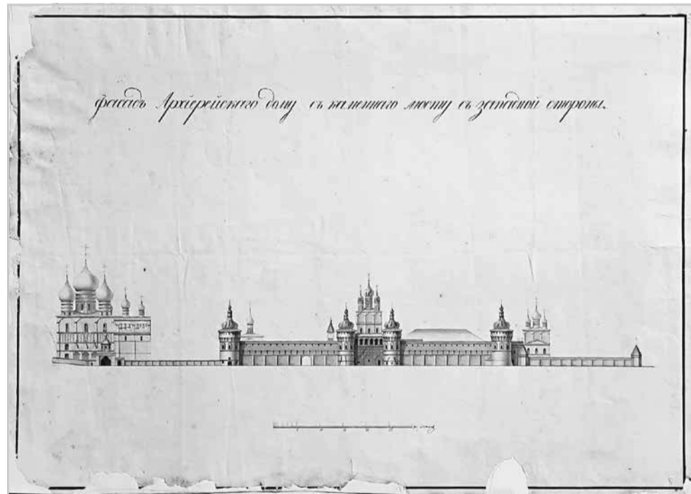
Ил. 3. Чертеж западного фасада Ростовского кремля. 1830-е гг. Копия с чертежа П. Я. Панькова 1818 г. ГМЗРК. АР-78
